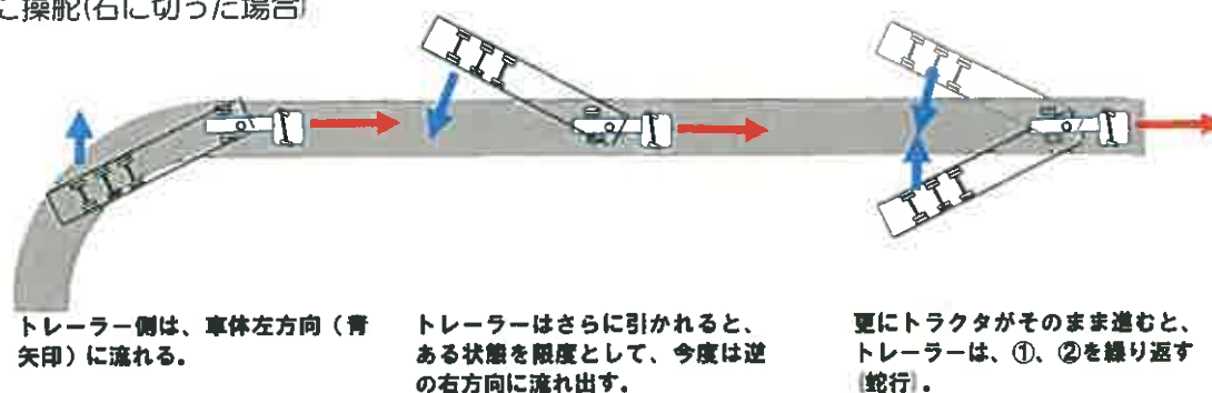
図9 トレーラーの蛇行
