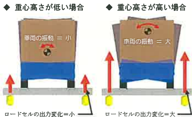
図4.3 重心高さの測定原理
